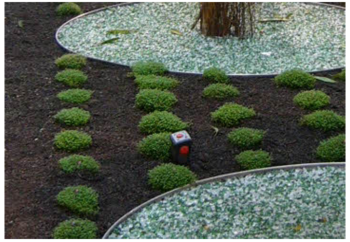
Bodenfeuchtesenor elektro-thermisch
